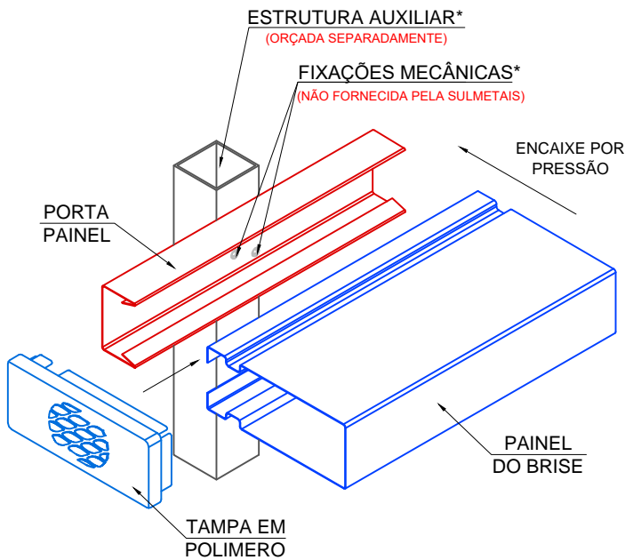
ESQUEMA DE MONTAGEM DO BRISE
