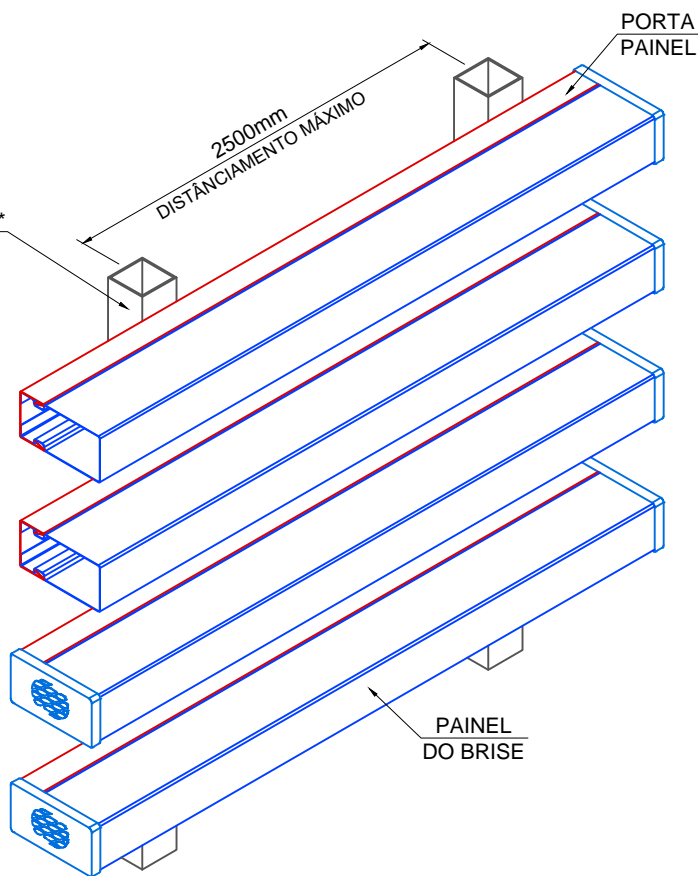
PERSPECTIVA DO BRISE
