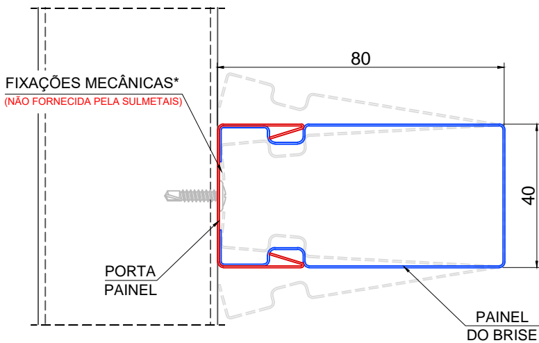
DETALHE DO PAINEL DO BRISE
