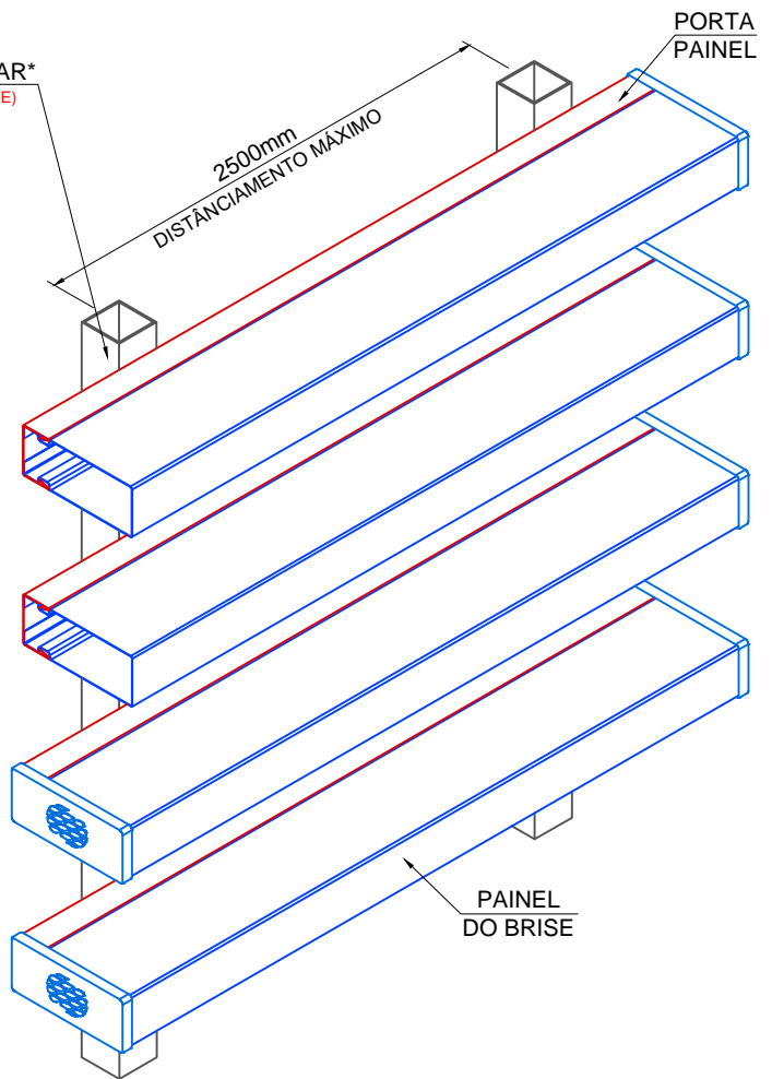
PERSPECTIVA DO BRISE
