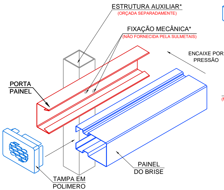
ESQUEMA DE MONTAGEM DO BRISE
