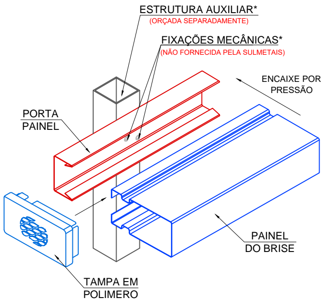
ESQUEMA DE MONTAGEM DO BRISE
