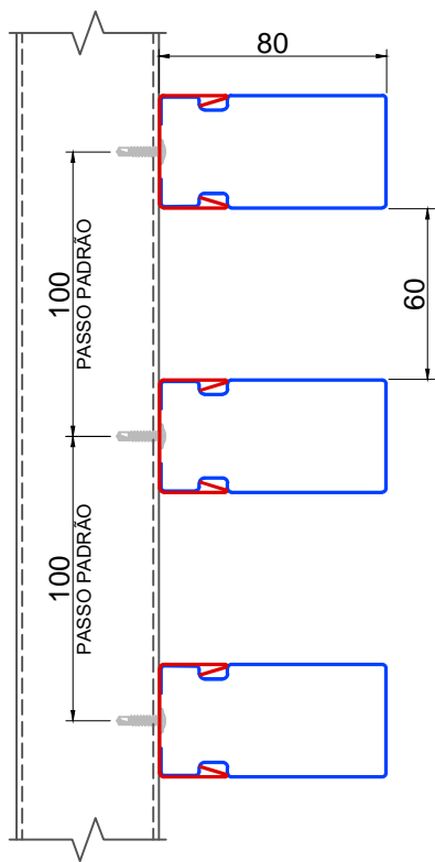
DETALHE DO BRISE
