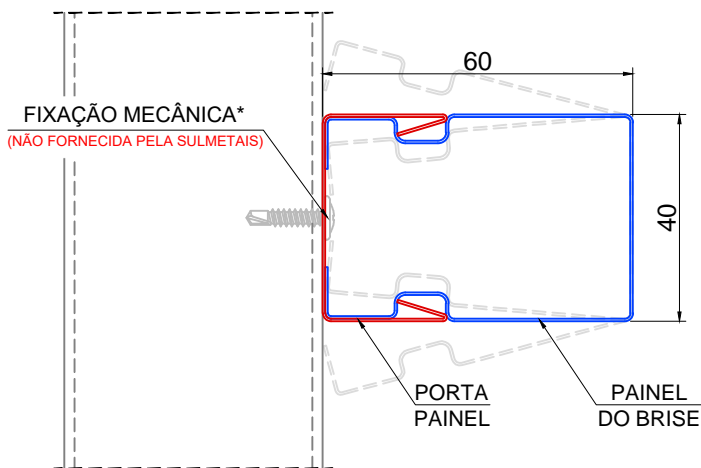
DETALHE DO PAINEL DO BRISE
