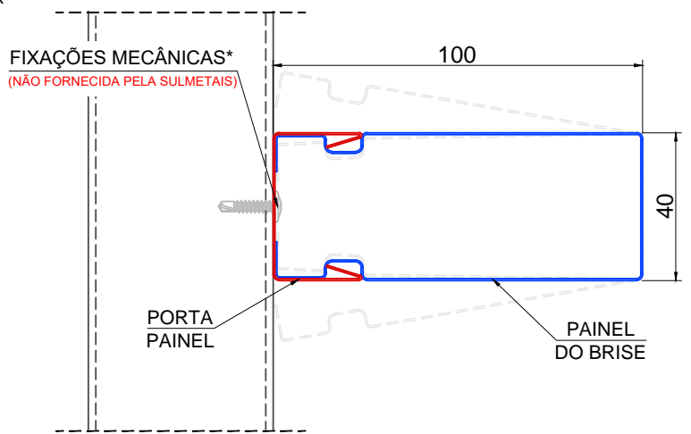
DETALHE DO PAINEL DO BRISE
