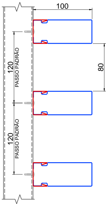
DETALHE DO BRISE
